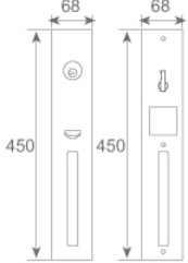
Size (尺寸圖) mm
