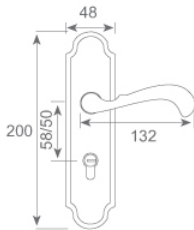
Size (尺寸圖) mm
