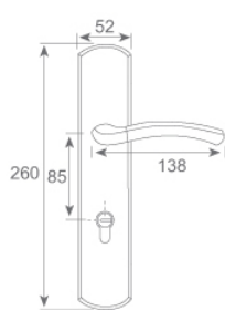
Size (尺寸圖) mm
