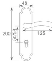
Size (尺寸圖) mm
