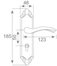
Size (尺寸圖) mm
