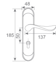
Size (尺寸圖) mm
