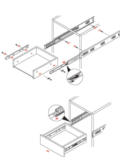
Installing Demonstration 安裝示範圖
