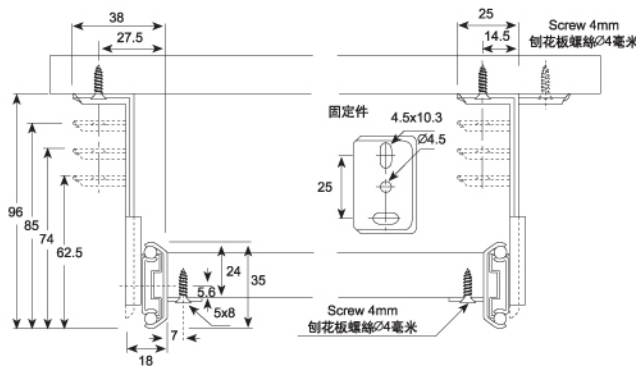
Install Dimension 安裝尺寸圖
