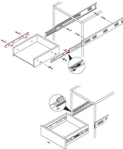
Installing Demonstration 安裝示範圖
