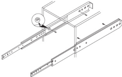
Installing Demonstration 安裝示範圖
