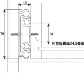
Install Dimension 安裝尺寸圖
