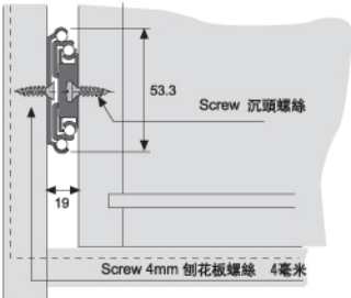
Install Dimension 安裝尺寸圖
