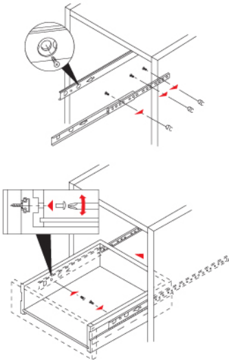
Installing Demonstration 安裝示範圖
