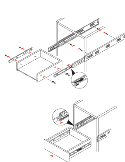
Installing Demonstration 安裝示範圖
