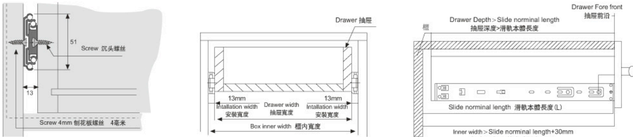
Install Dimension 安裝尺寸圖
