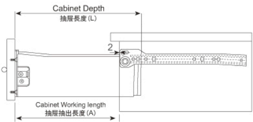
Stop Position 抽屜拉出停止位置
