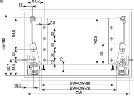
Installation Dimension 安裝尺寸圖
