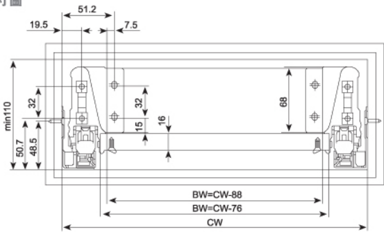
Installation Dimension 安裝尺寸圖
