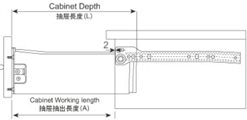
Stop Position 抽屜拉出停止位置
