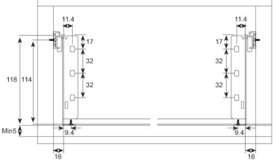
Installation Dimension 固定軌安裝孔位
