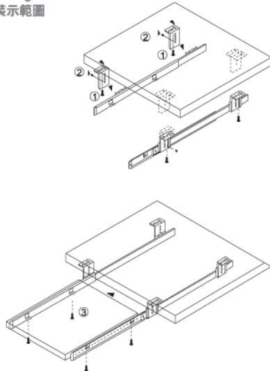
Installing Demonstration 安裝示範圖
