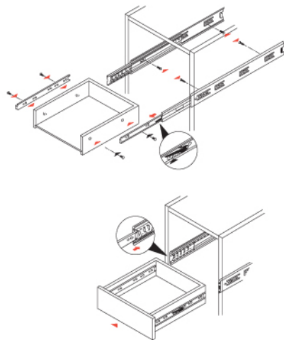
Installing Demonstration 安裝示範圖
