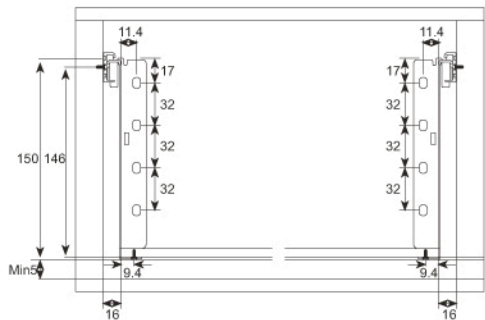
Installation Dimension 固定軌安裝孔位
