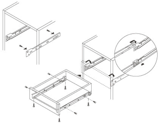
Installing Demonstration 安裝示範圖
