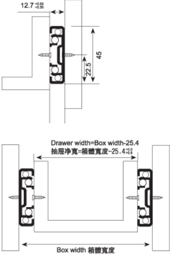
Install Dimension 安裝尺寸圖
