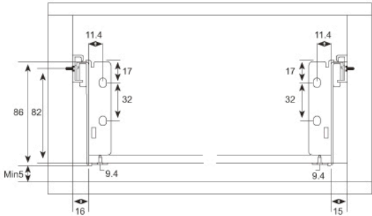
Installation Dimension 固定軌安裝孔位
