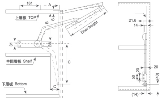
Installation indication 安裝孔位示意圖
