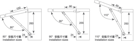
Installation indication 安裝孔位示意圖
