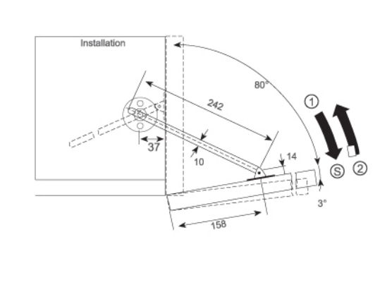
Installation indication 安裝孔位示意圖
