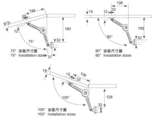
Installation indication 安裝孔位示意圖
