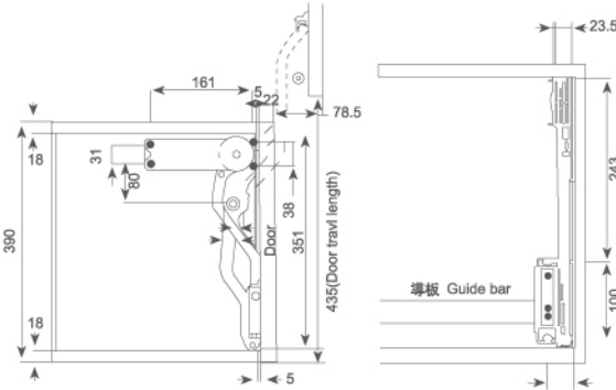
Installation indication 安裝孔位示意圖
