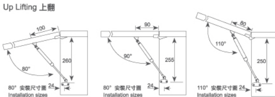
Installation indication 安裝孔位示意圖
